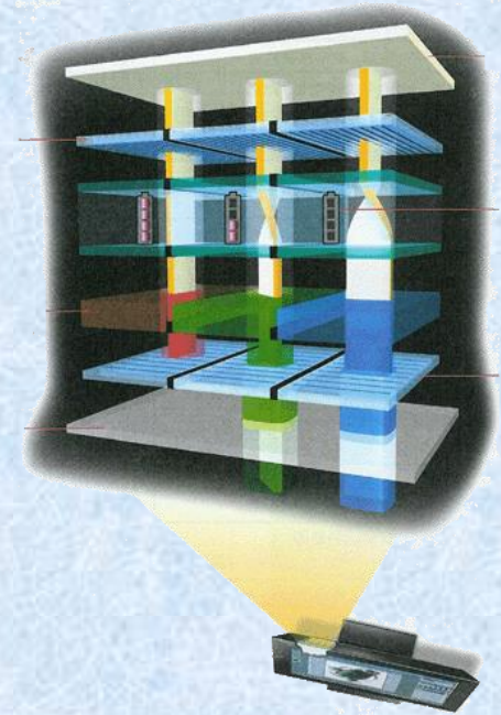
Folyadékkristályos kijelző (LCD) működése
