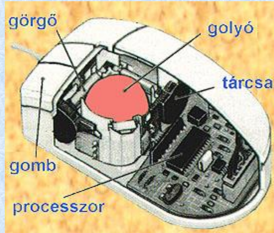
Golyós egér felépítése
